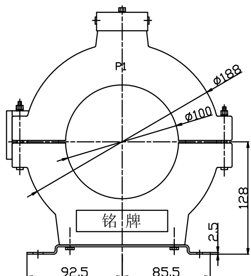
外形尺寸图 Overall dimensions
