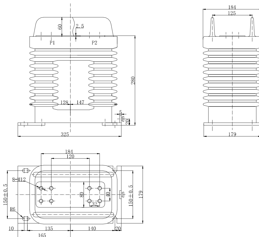
外形尺寸图 Overall dimensions
