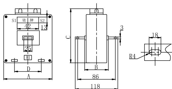
LZK-0.66I 出排式 示意图
