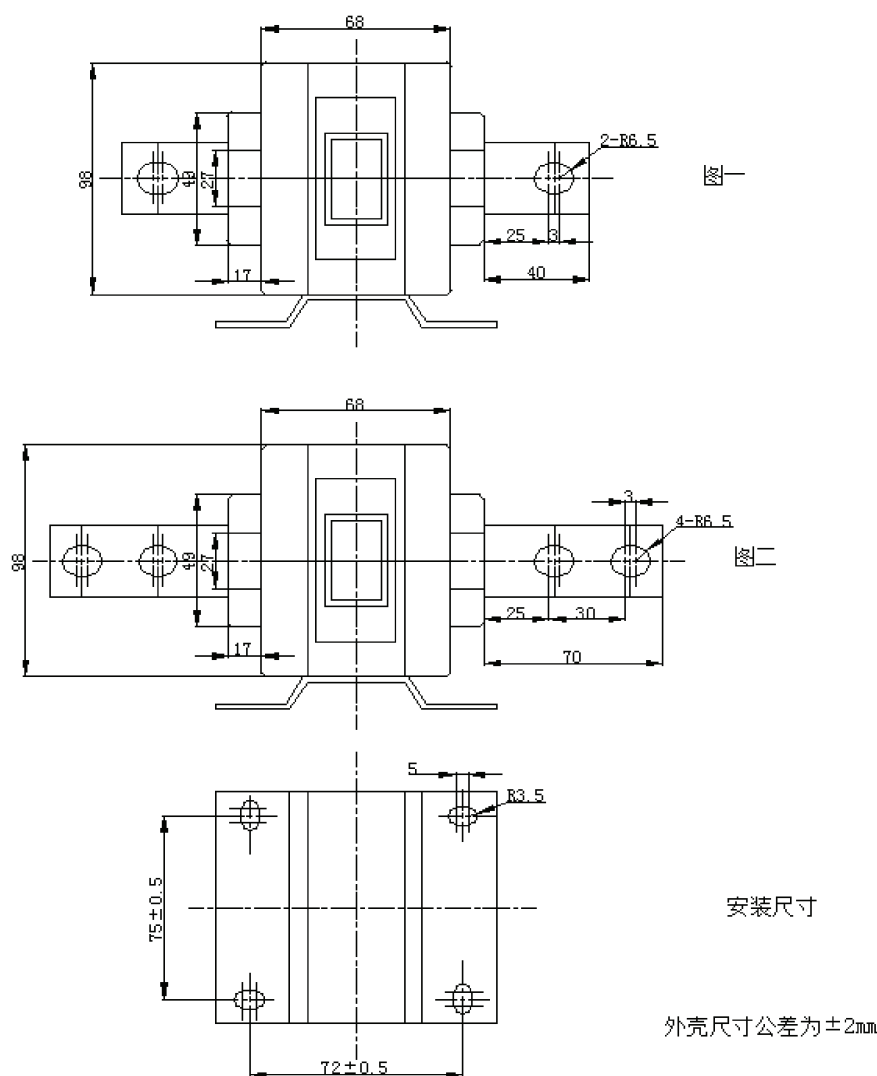
外形尺寸图 Overall dimensions
