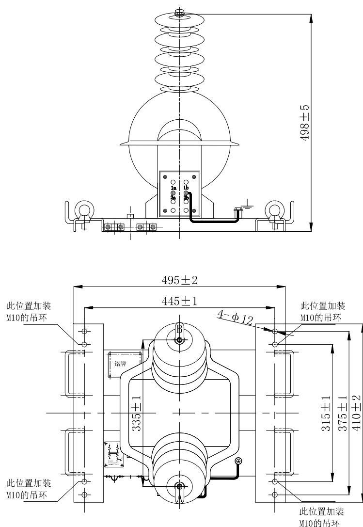
外形尺寸图 Overall dimensions
