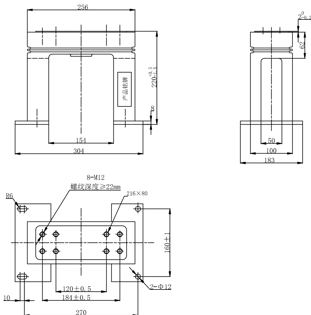
外形尺寸图 Overall dimensions
