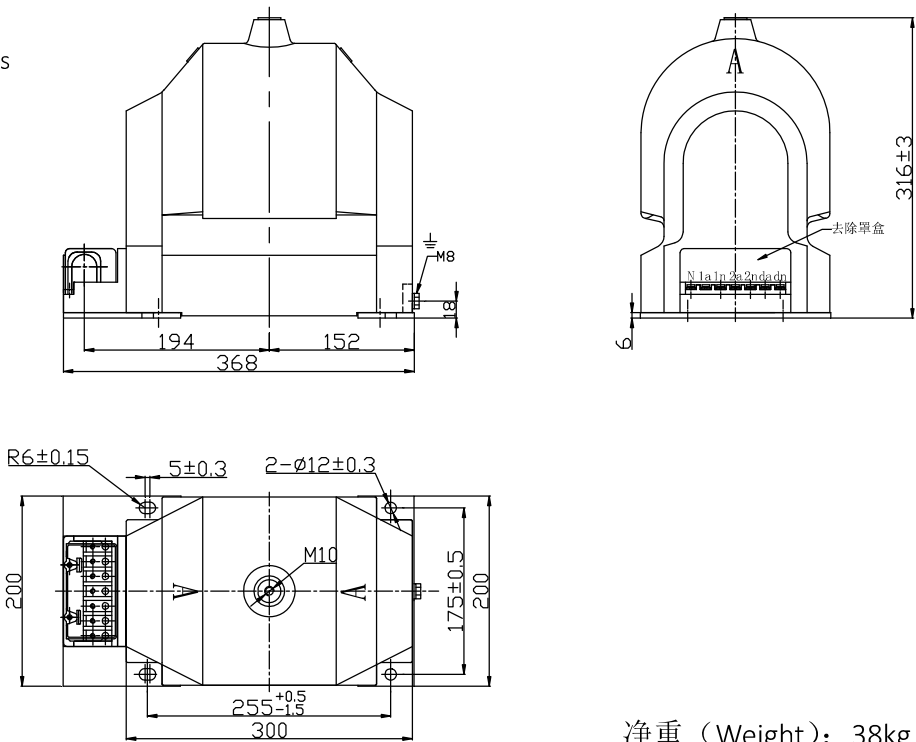
外形尺寸图
