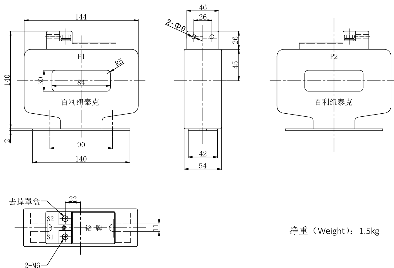
外形尺寸图 Overall dimensions
