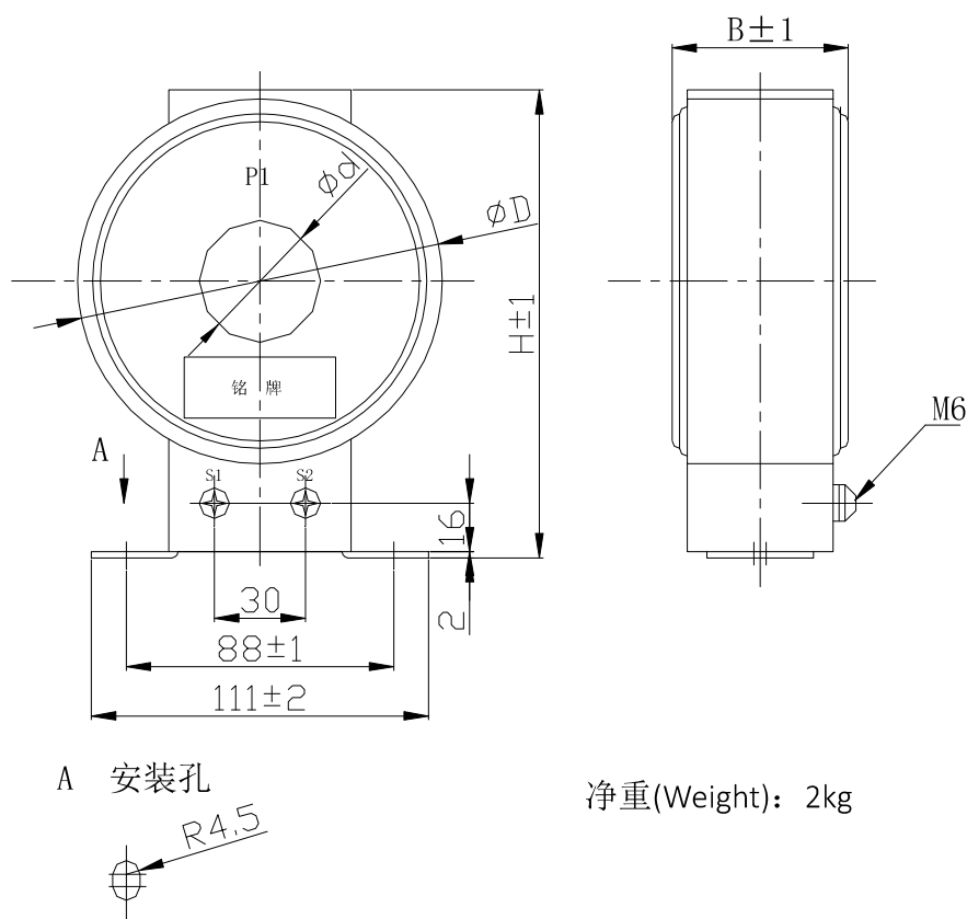
外形尺寸图 Overall dimensions
