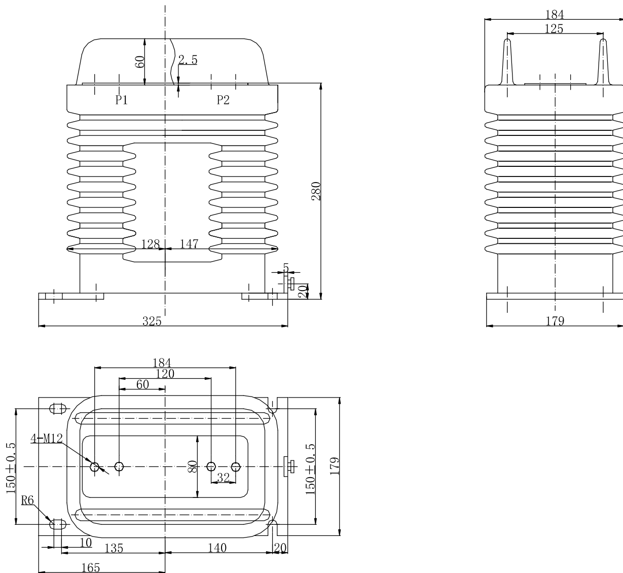
外形尺寸图 Overall dimensions
