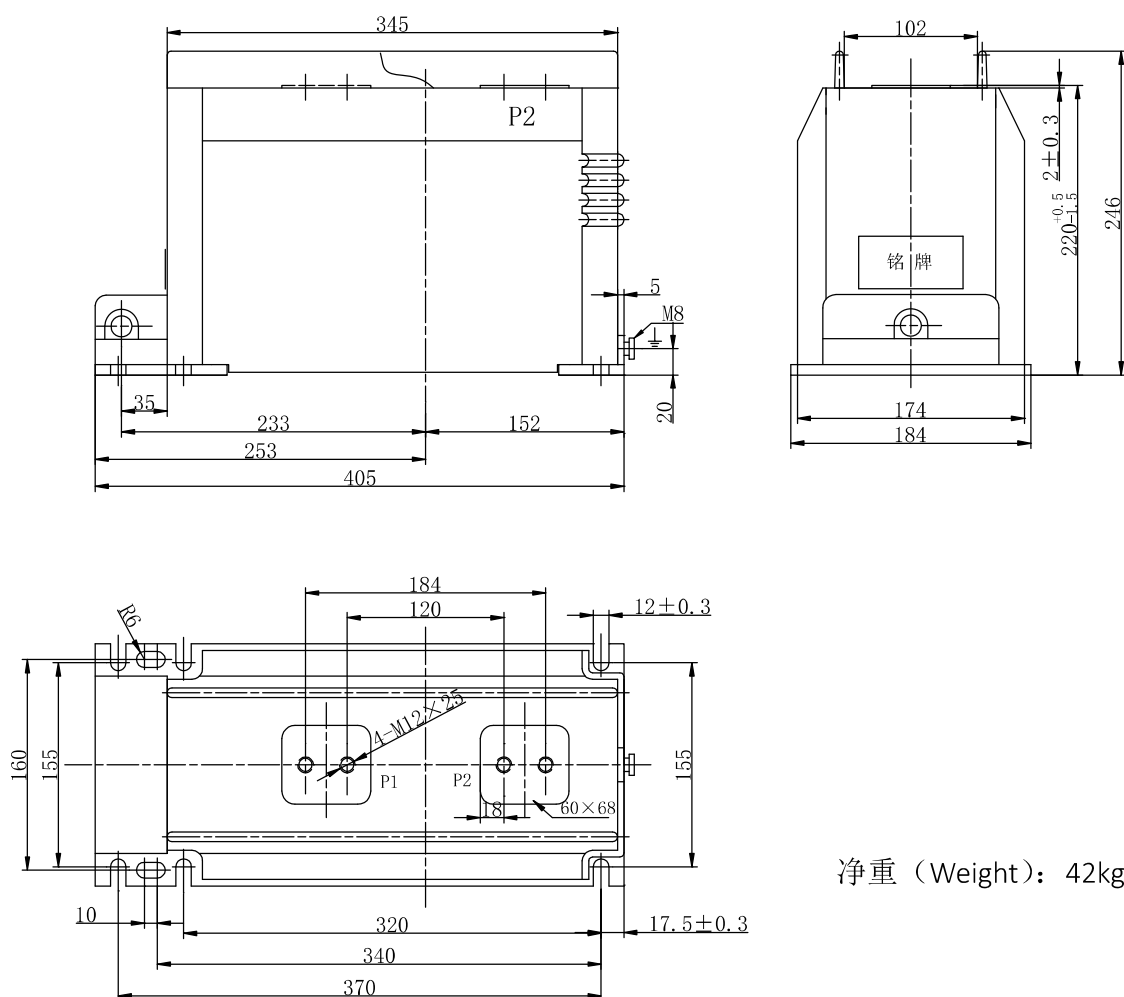
外形尺寸图 Overall dimensions
