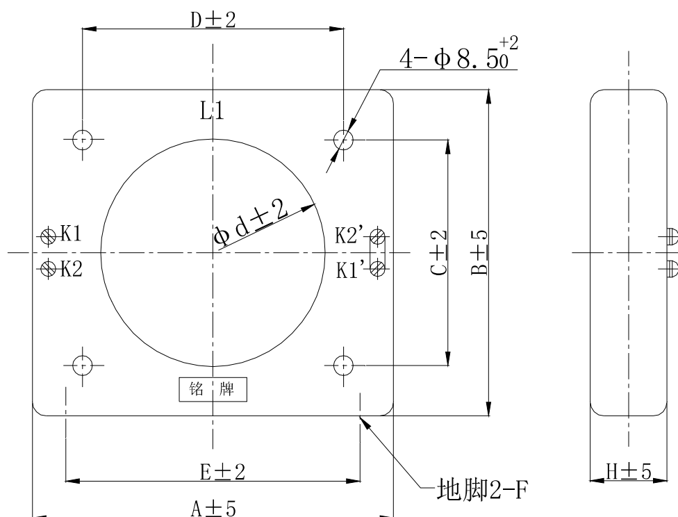
外形尺寸图 Overall dimensions
