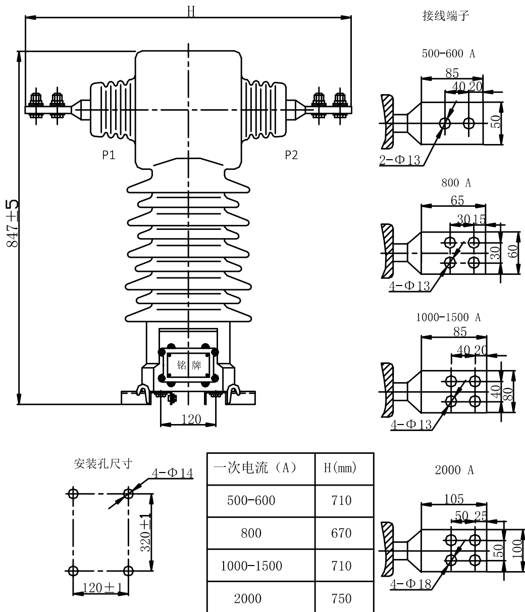
外形尺寸图 Overall dimensions
