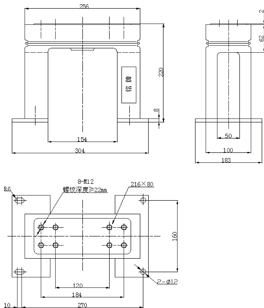
外形尺寸图 Overall dimensions
