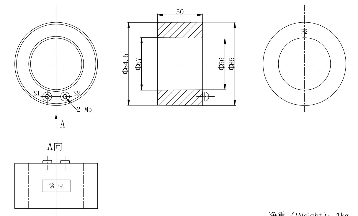
外形尺寸图 Overall dimensions
