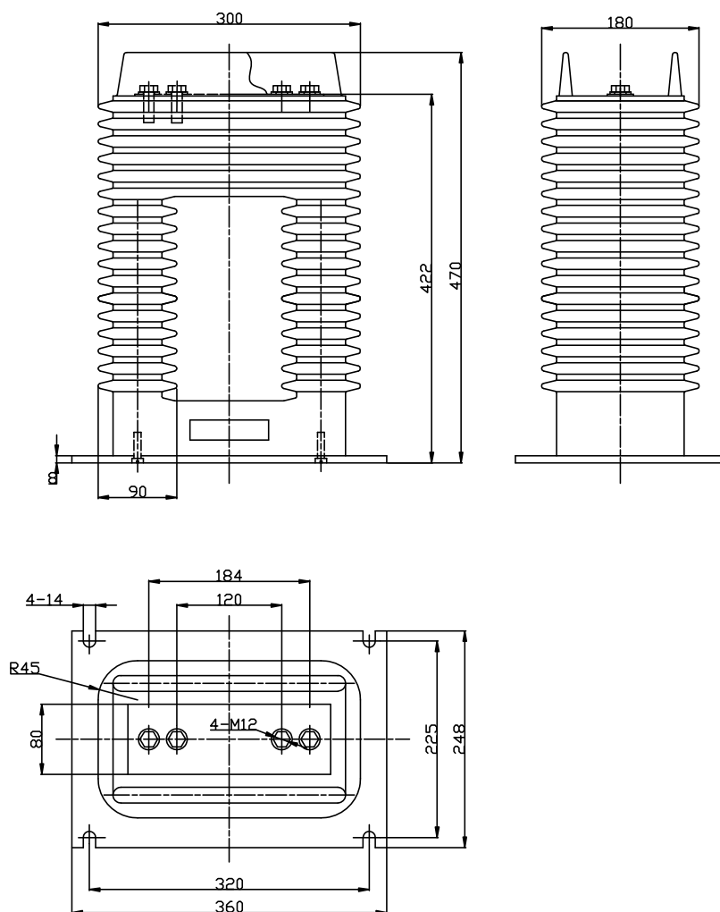
外形尺寸图 Overall dimensions
