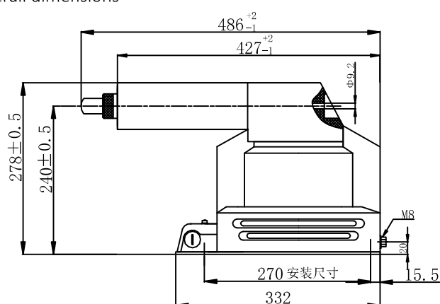
外形尺寸图
