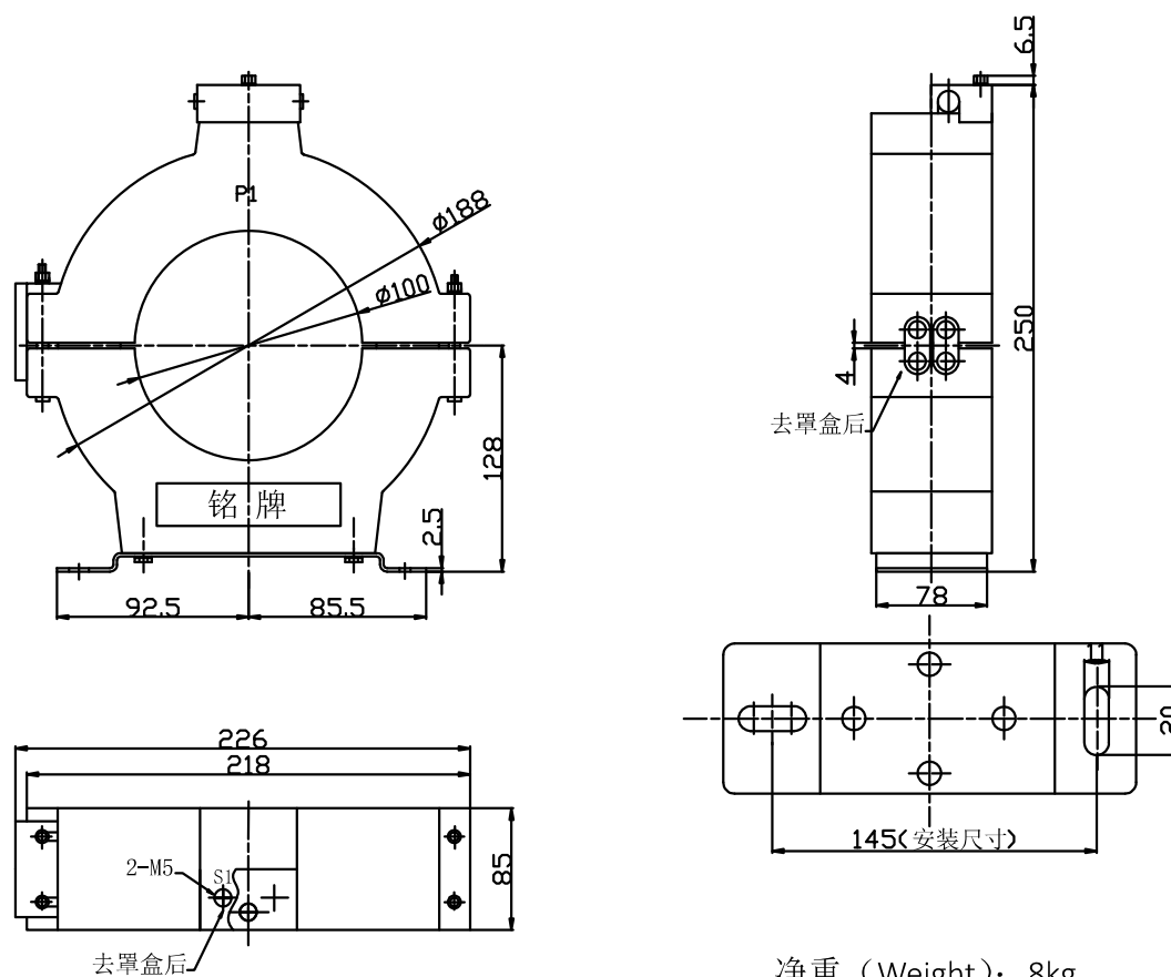
外形尺寸图 Overall dimensions
