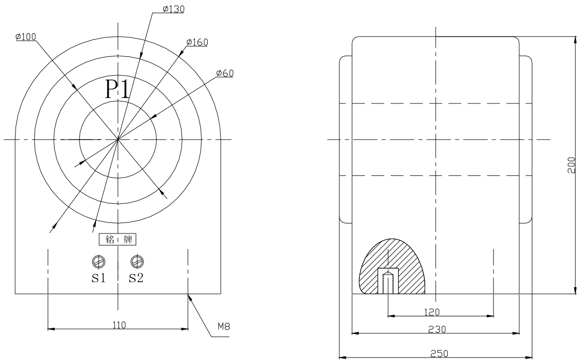
外形尺寸图 Overall dimensions
