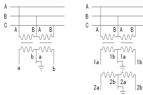
接线图 Wiring diagram
