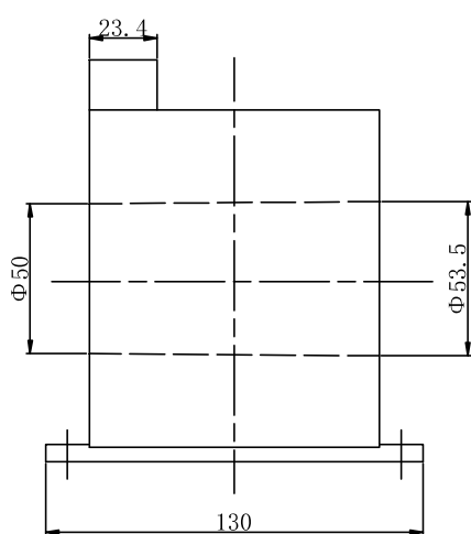
外形尺寸图 Overall dimensions
