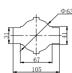
LZK-0.66I \Phi 100
