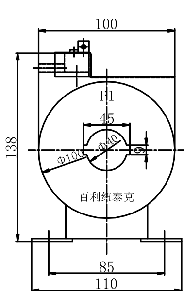
外形尺寸图 Overall dimensions
