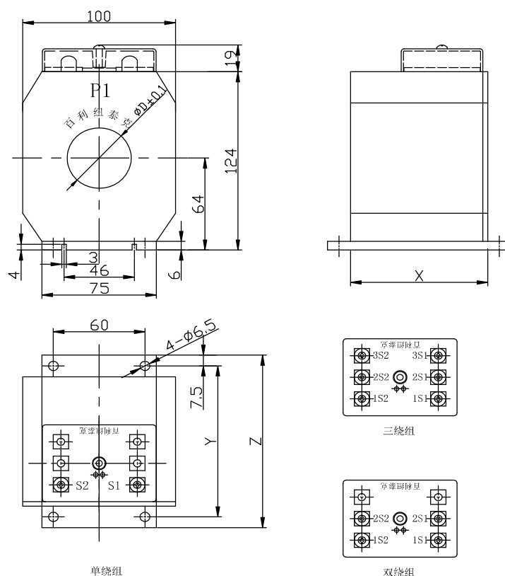
外形尺寸图 Overall dimensions
