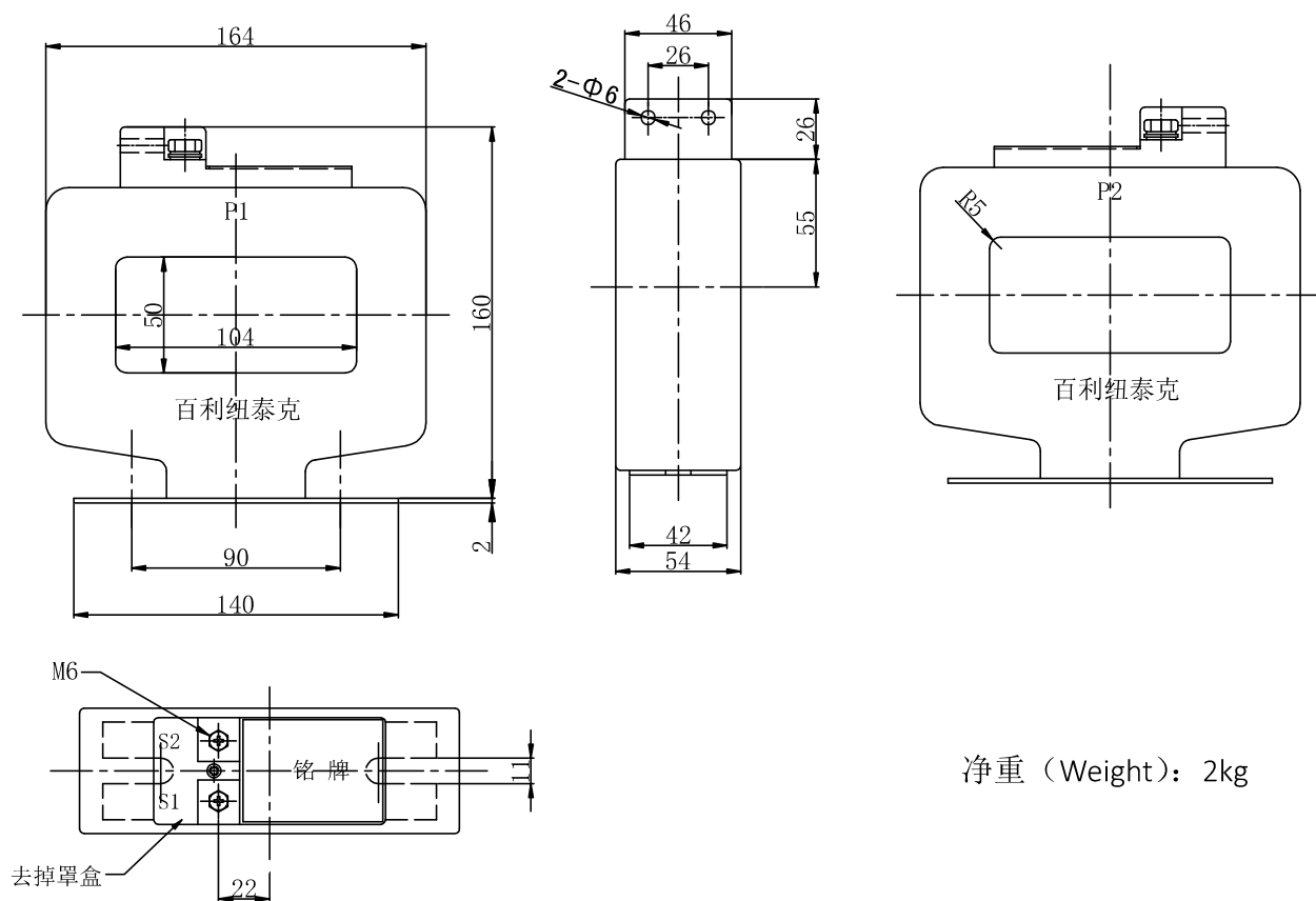
外形尺寸图 Overall dimensions
