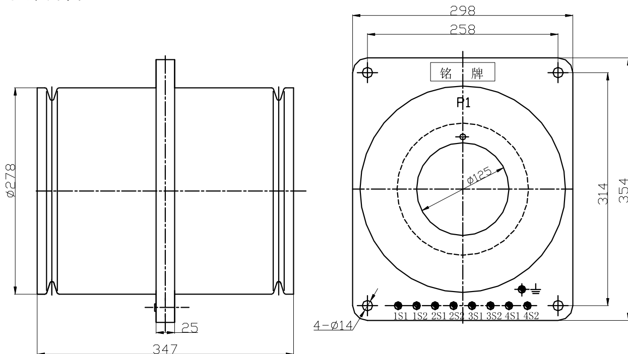
外形尺寸图 Overall dimensions
