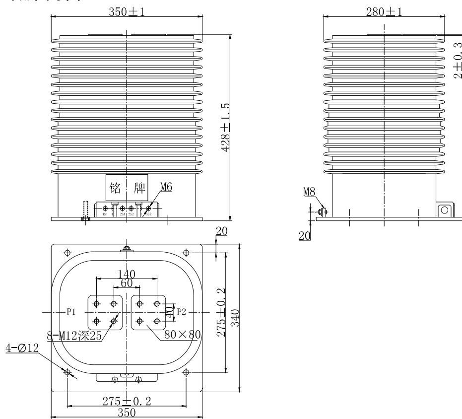
外形尺寸图 Overall dimensions
