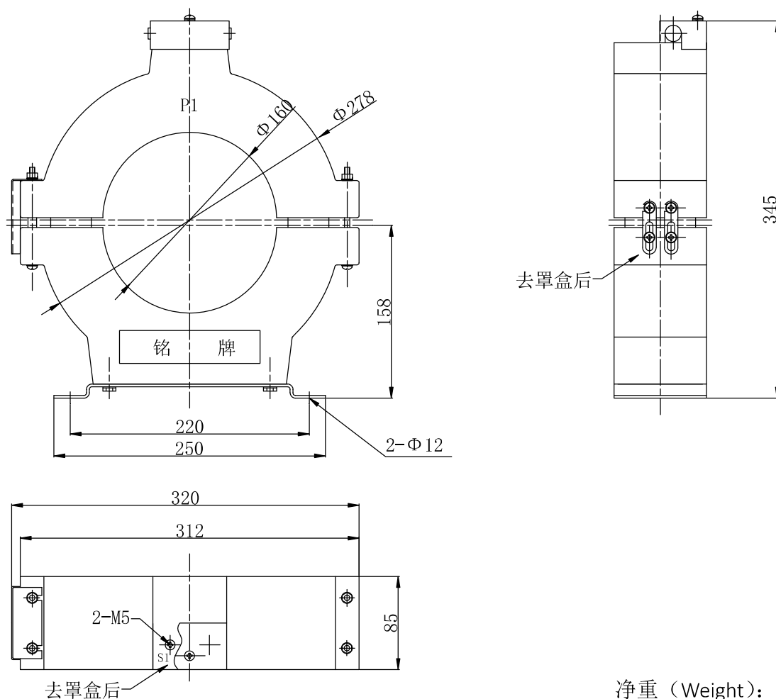
外形尺寸图 Overall dimensions
