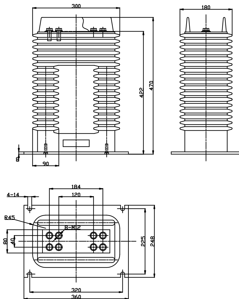
外形尺寸图 Overall dimensions
