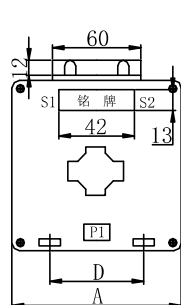
LZK-0.66I 穿心式 示意图
