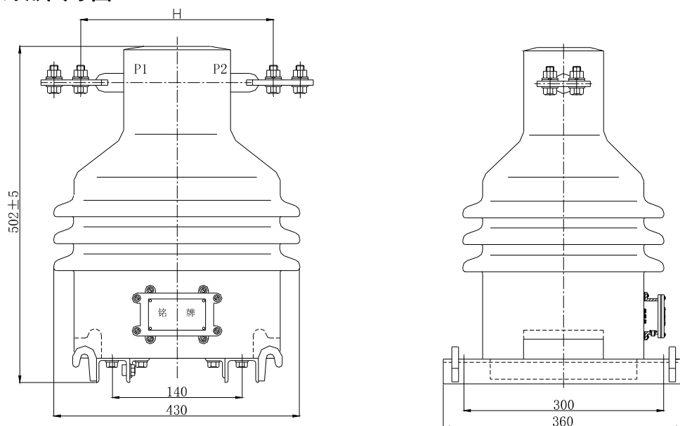
安装孔尺寸
