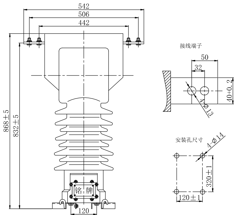
外形尺寸图 Overall dimensions
