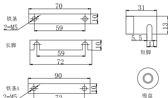
配件示意图
