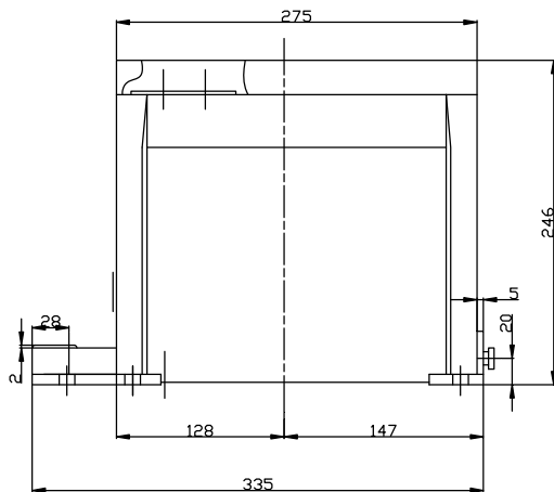
外形尺寸图 Overall dimensions
