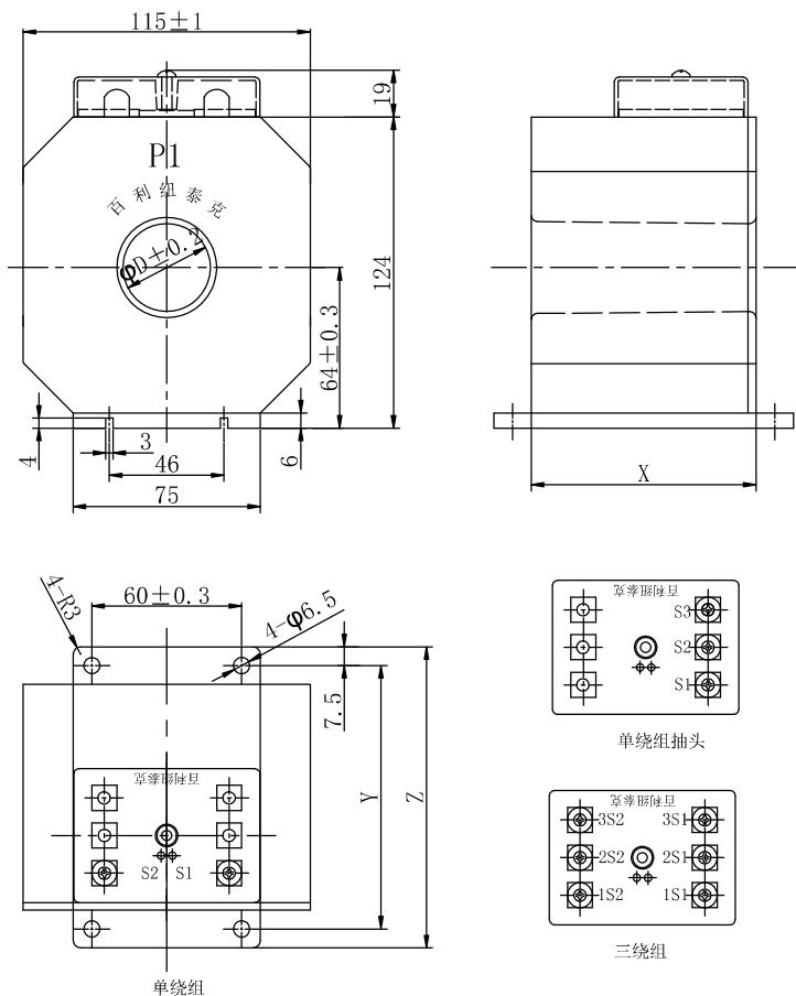
外形尺寸图 Overall dimensions
