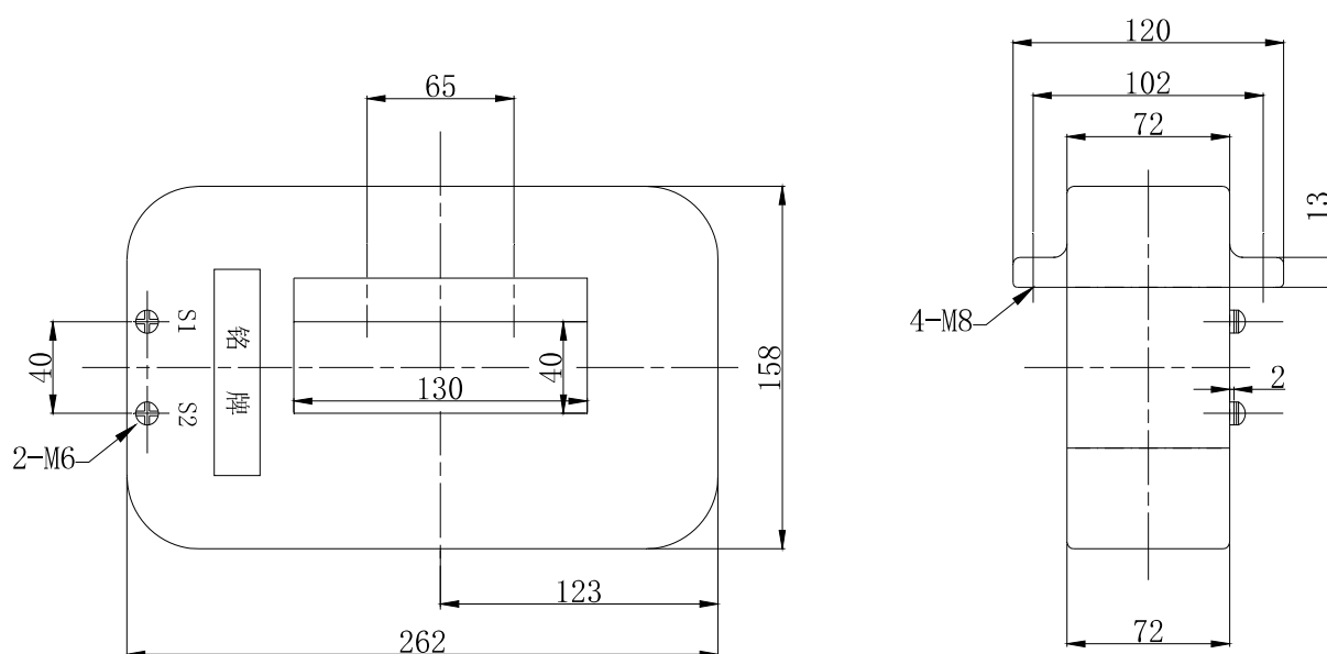
外形尺寸图 Overall dimensions
