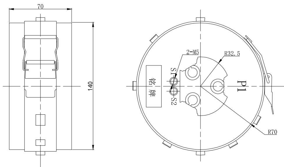
外形尺寸图 Overall dimensions
