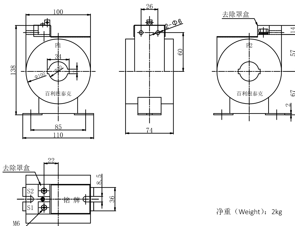
外形尺寸图 Overall dimensions
