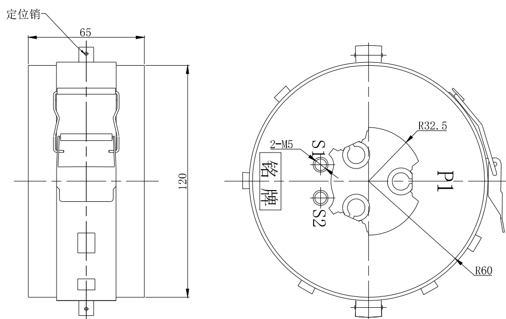
外形尺寸图 Overall dimensions
