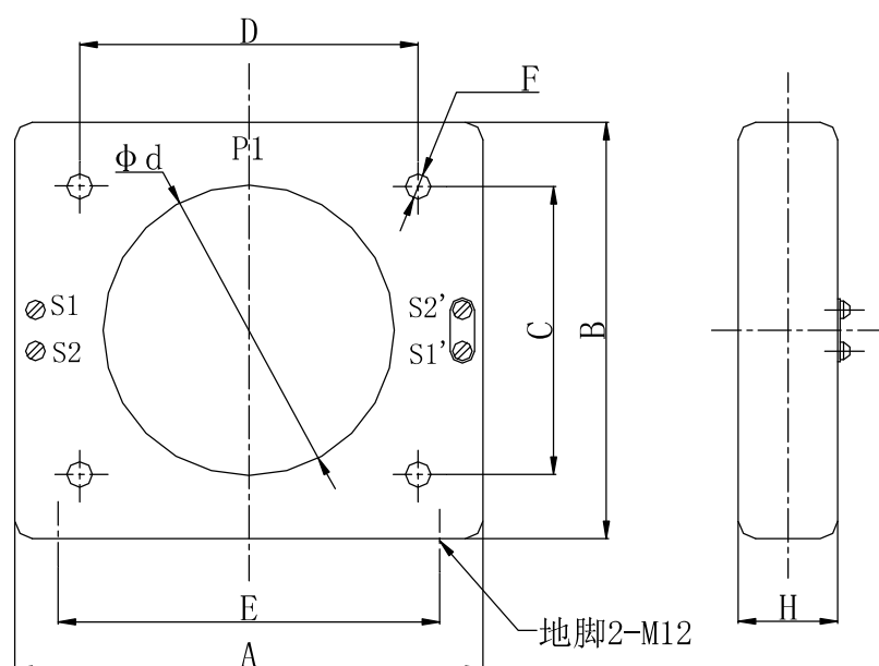
外形尺寸图 Overall dimensions
