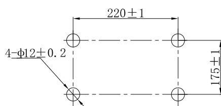
安装孔尺寸:
