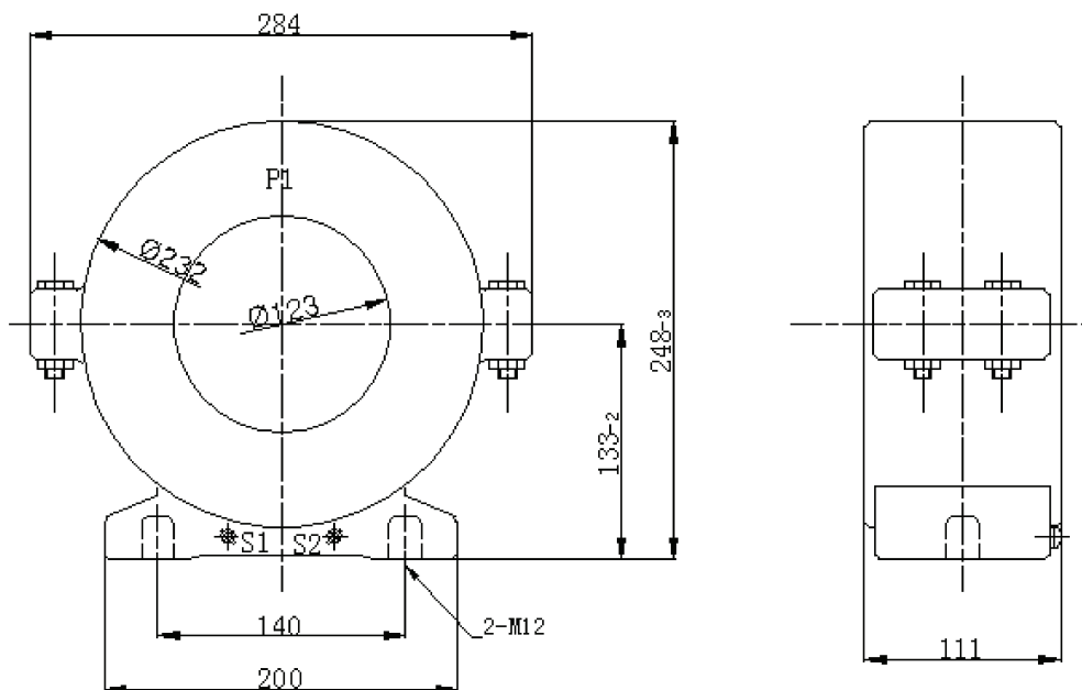
外形尺寸图 Overall dimensions
