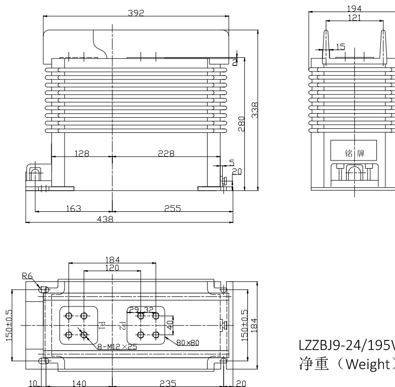
外形尺寸图 Overall dimensions
