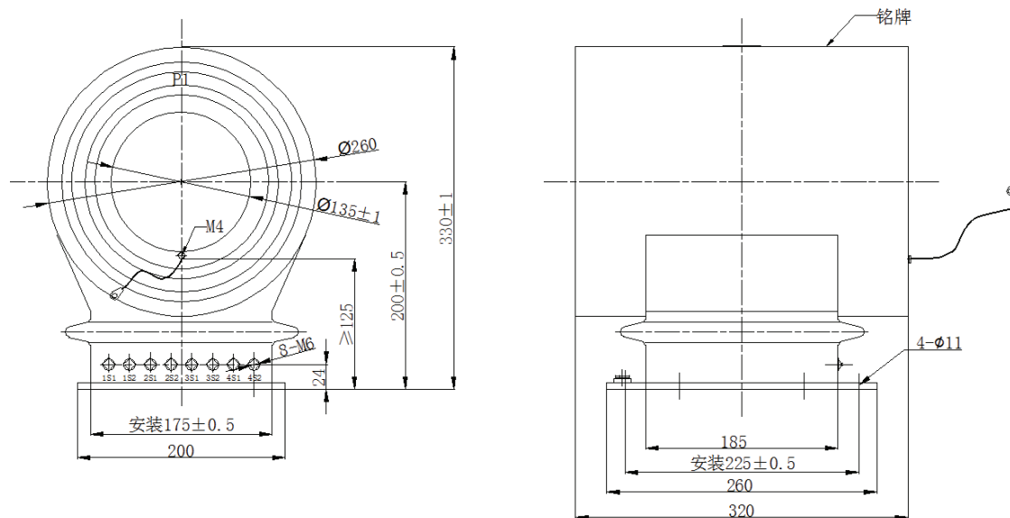
外形尺寸图 Overall dimensions
