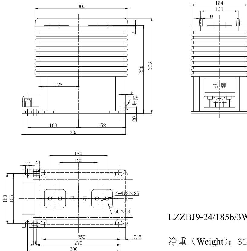
外形尺寸图 Overall dimensions
