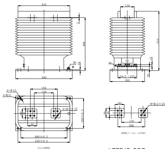
外形尺寸图 Overall dimensions
