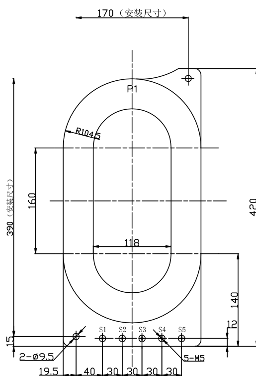
外形尺寸图 Overall dimensions
