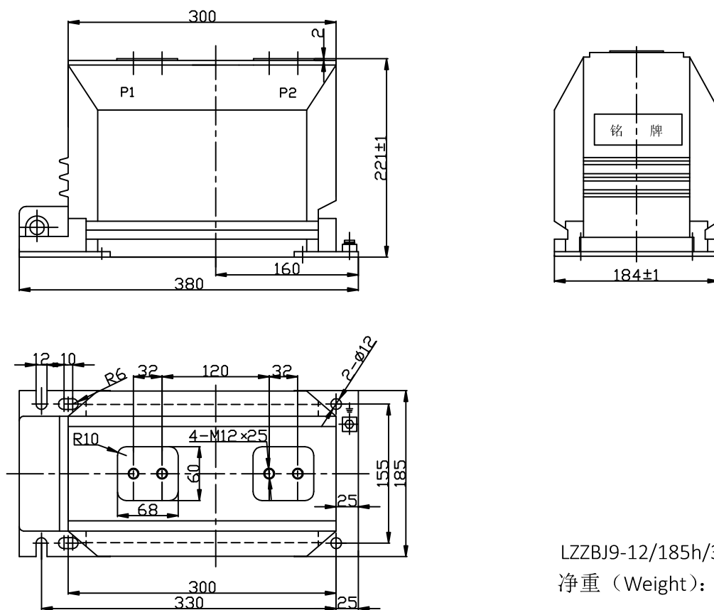
外形尺寸图 Overall dimensions
