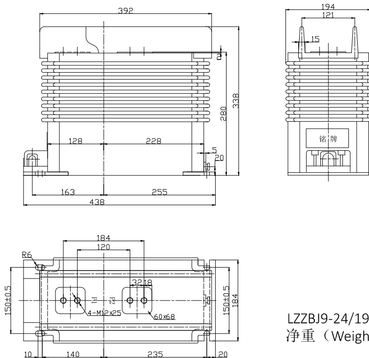
外形尺寸图 Overall dimensions
