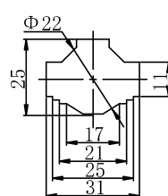
LZK-0.66I \Phi 30
