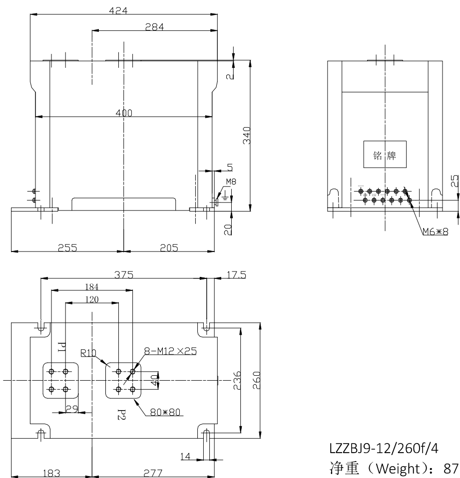
外形尺寸图 Overall dimensions
