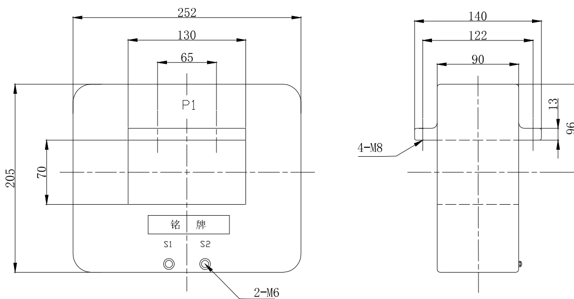
外形尺寸图 Overall dimensions
