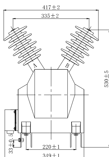
安装孔尺寸:
