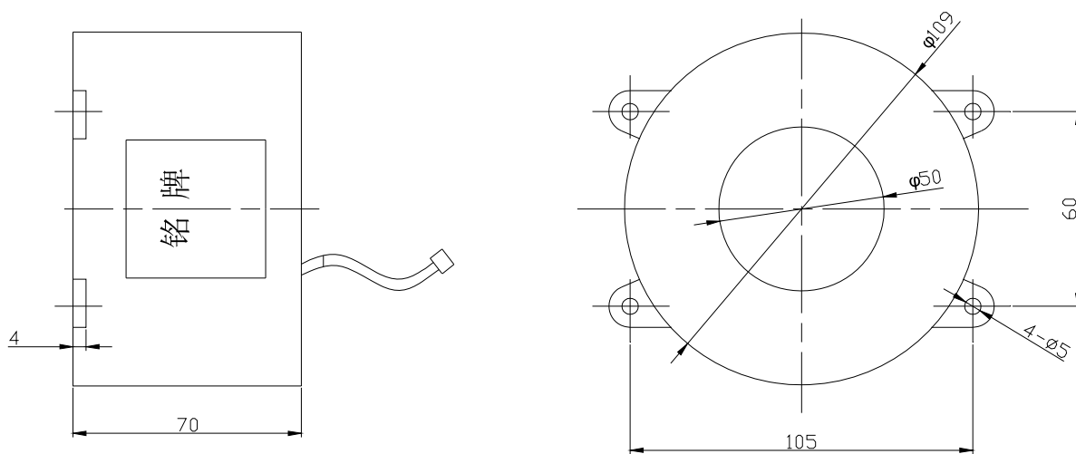
外形尺寸图 Overall dimensions
