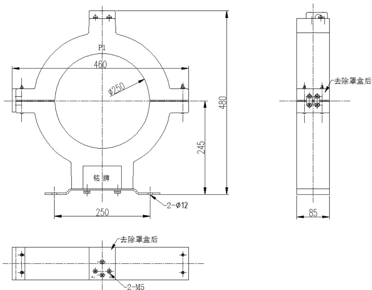
外形尺寸图 Overall dimensions
