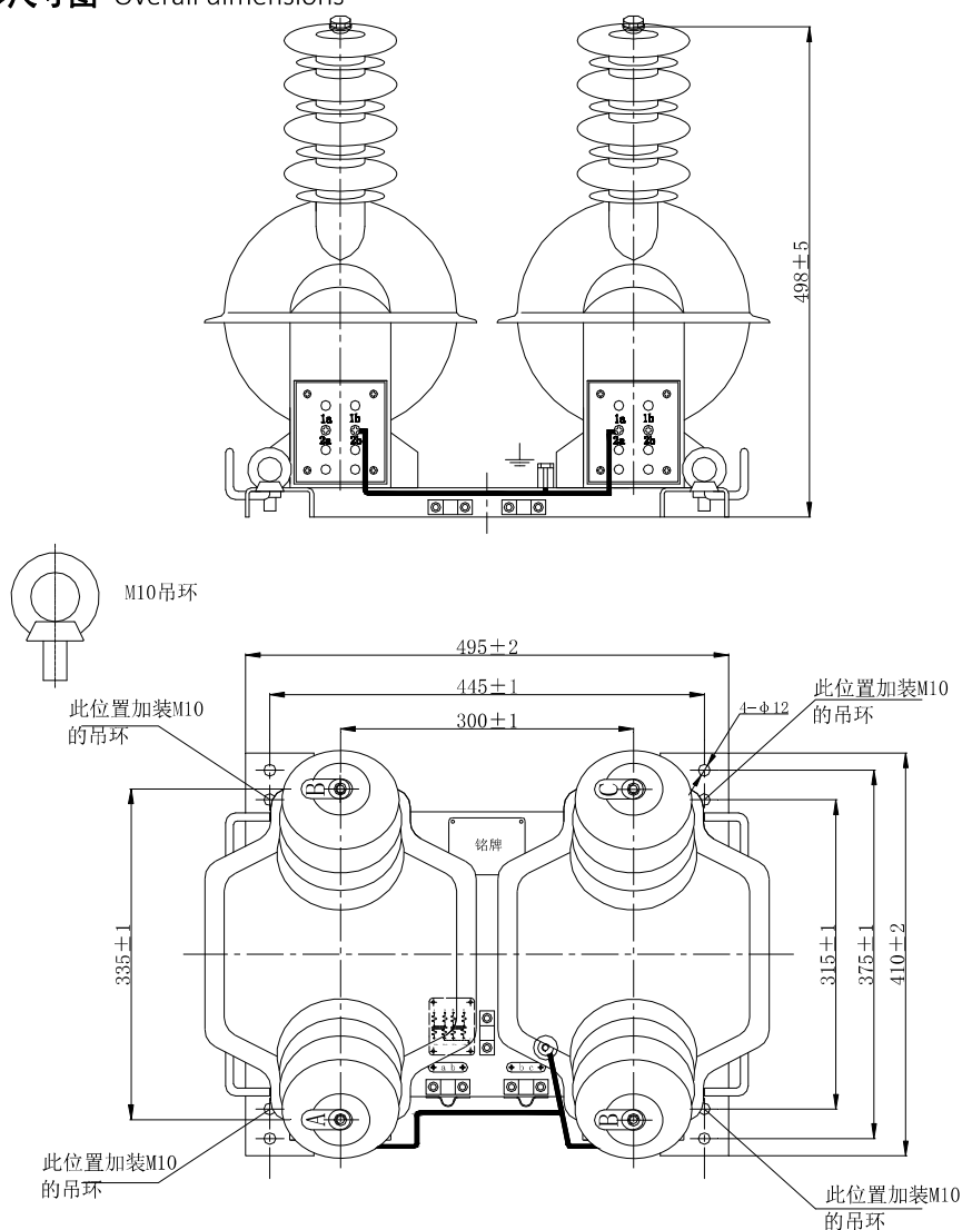
外形尺寸图 Overall dimensions
