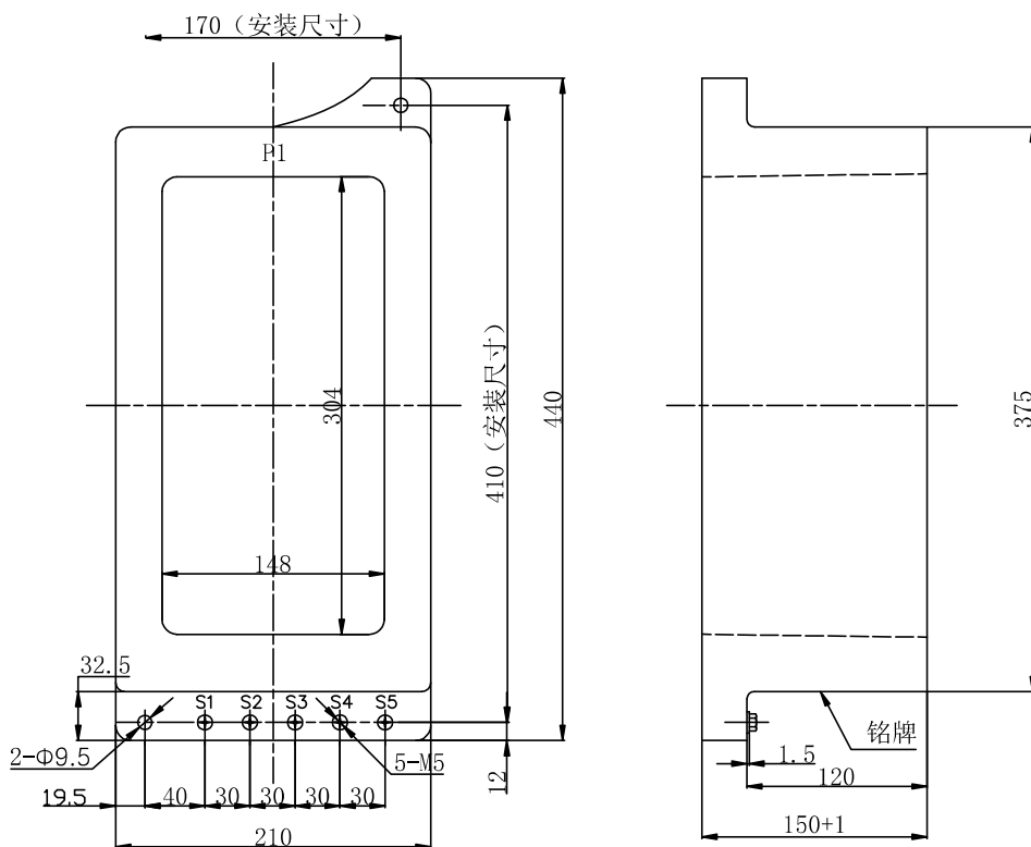
外形尺寸图 Overall dimensions
