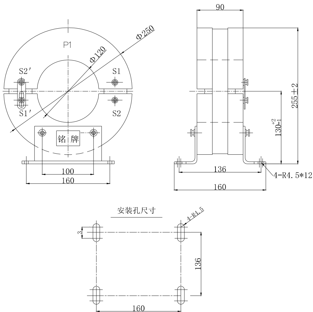
外形尺寸图 Overall dimensions
