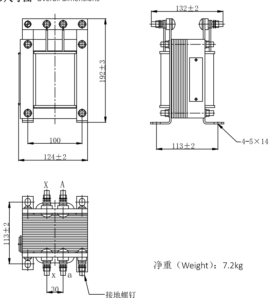
外形尺寸图 Overall dimensions
