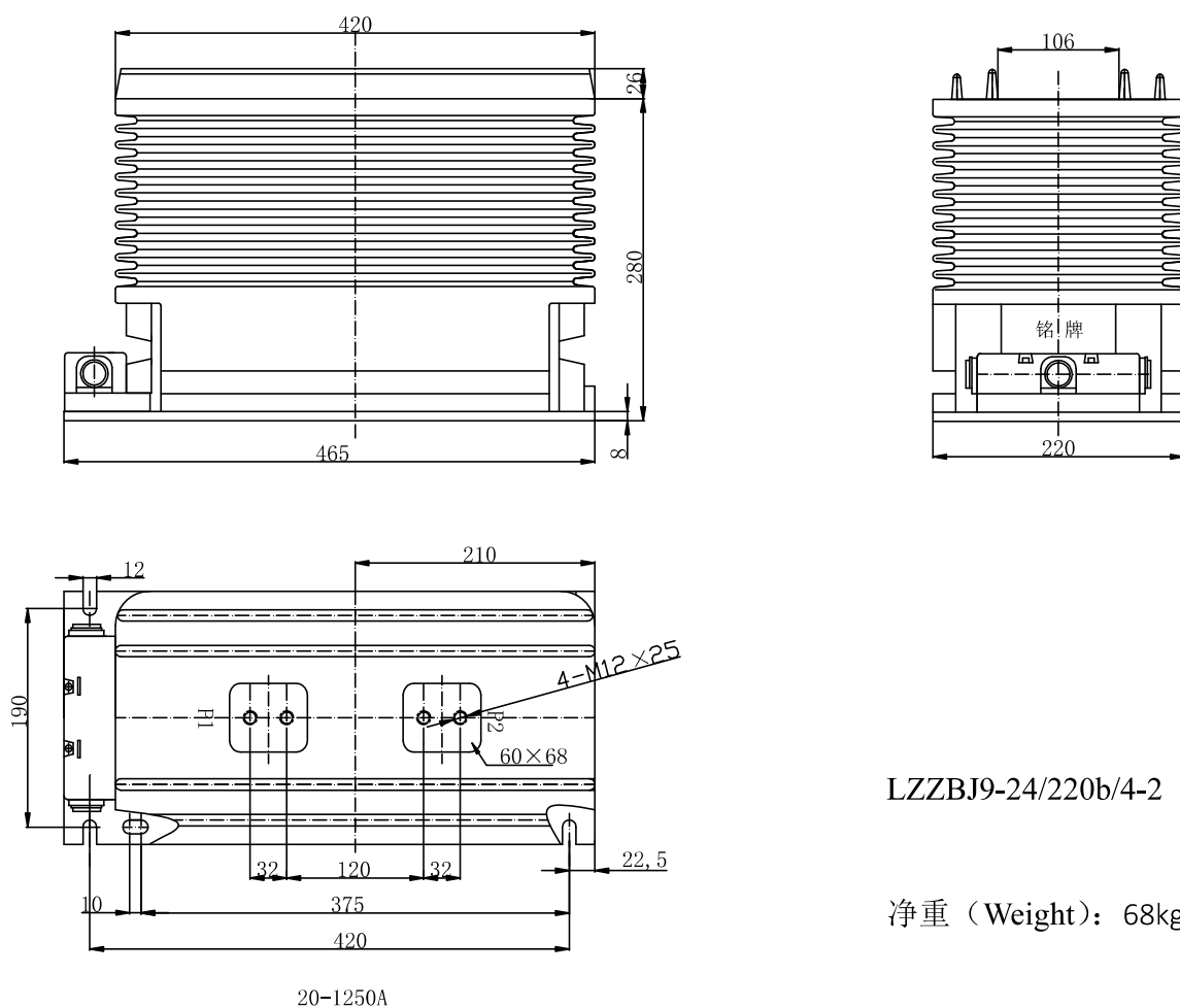
外形尺寸图 Overall dimensions
