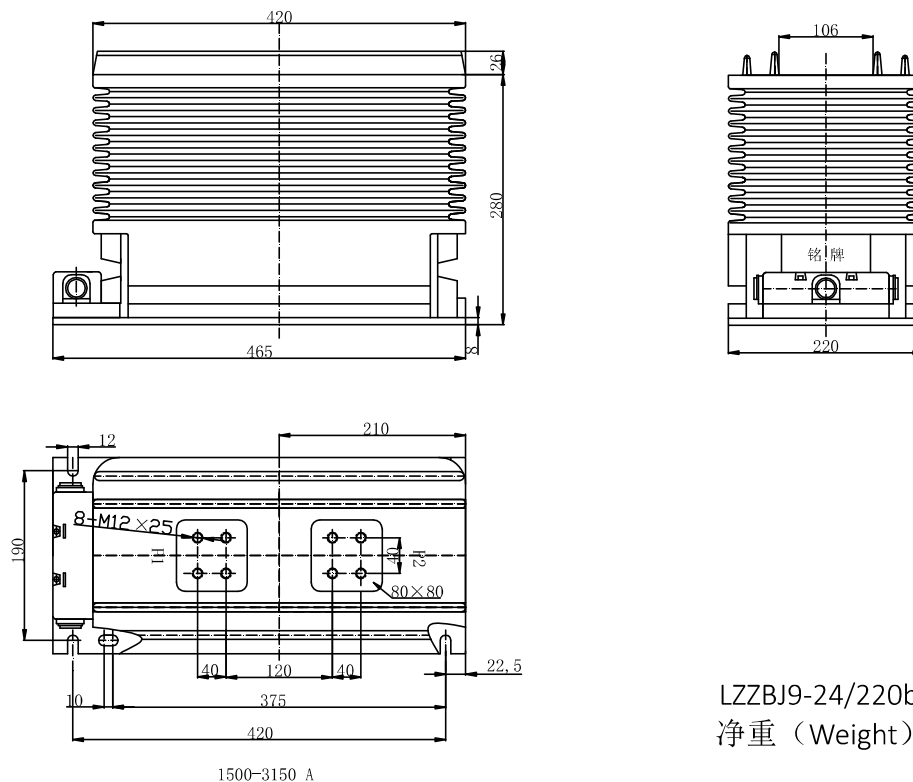
外形尺寸图 Overall dimensions
