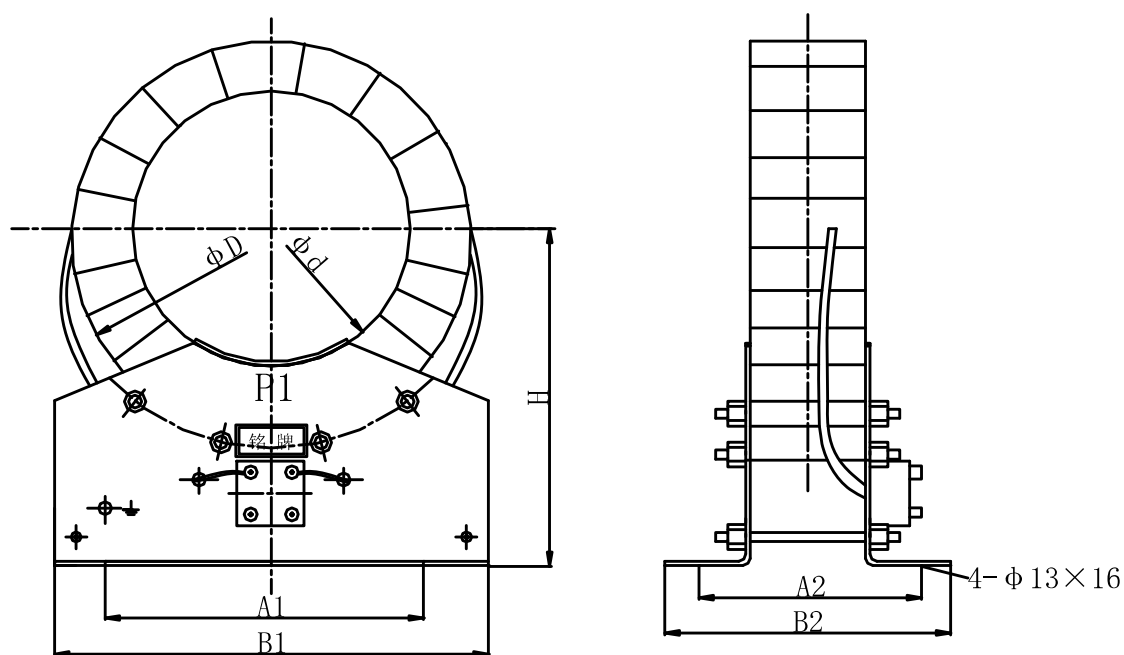
外形尺寸图 Overall dimensions
